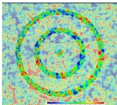
Círculos concéntricos en la radiación de fondo de microondas que indican un universo anterior. WMAP
